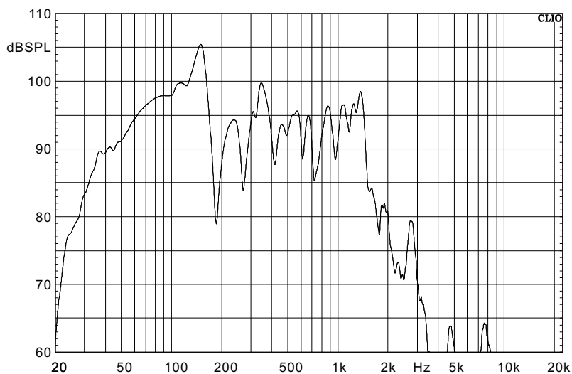
頻響曲綫
